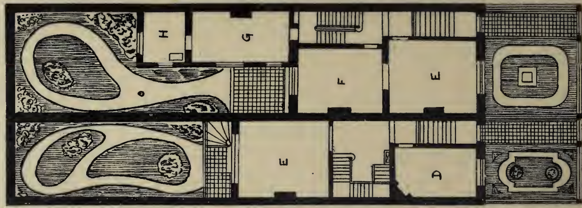
REZ DE CHAUSSÉE.
